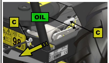
Obr. 13: Spojka pojezdu
