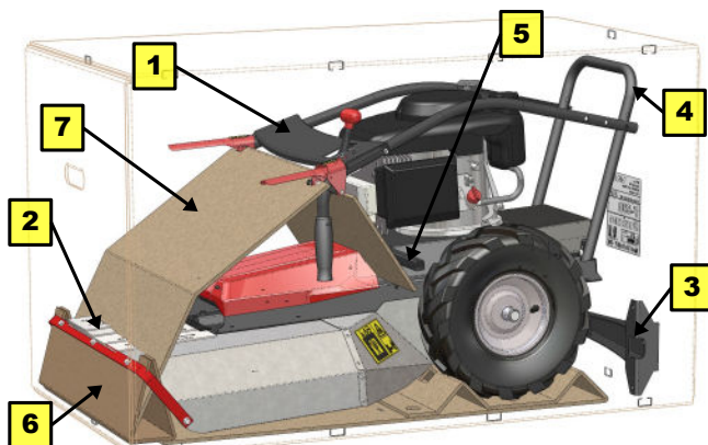
Obr. 1: Vybalení stroje
