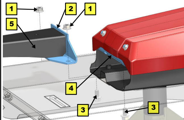
Obr. 2: Sestavení stroje
